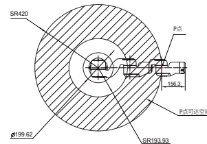
JAKA MiniCobo P点可达空间正视(上)俯视(下)
