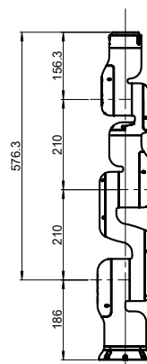
JAKA MiniCobo外形尺寸图
